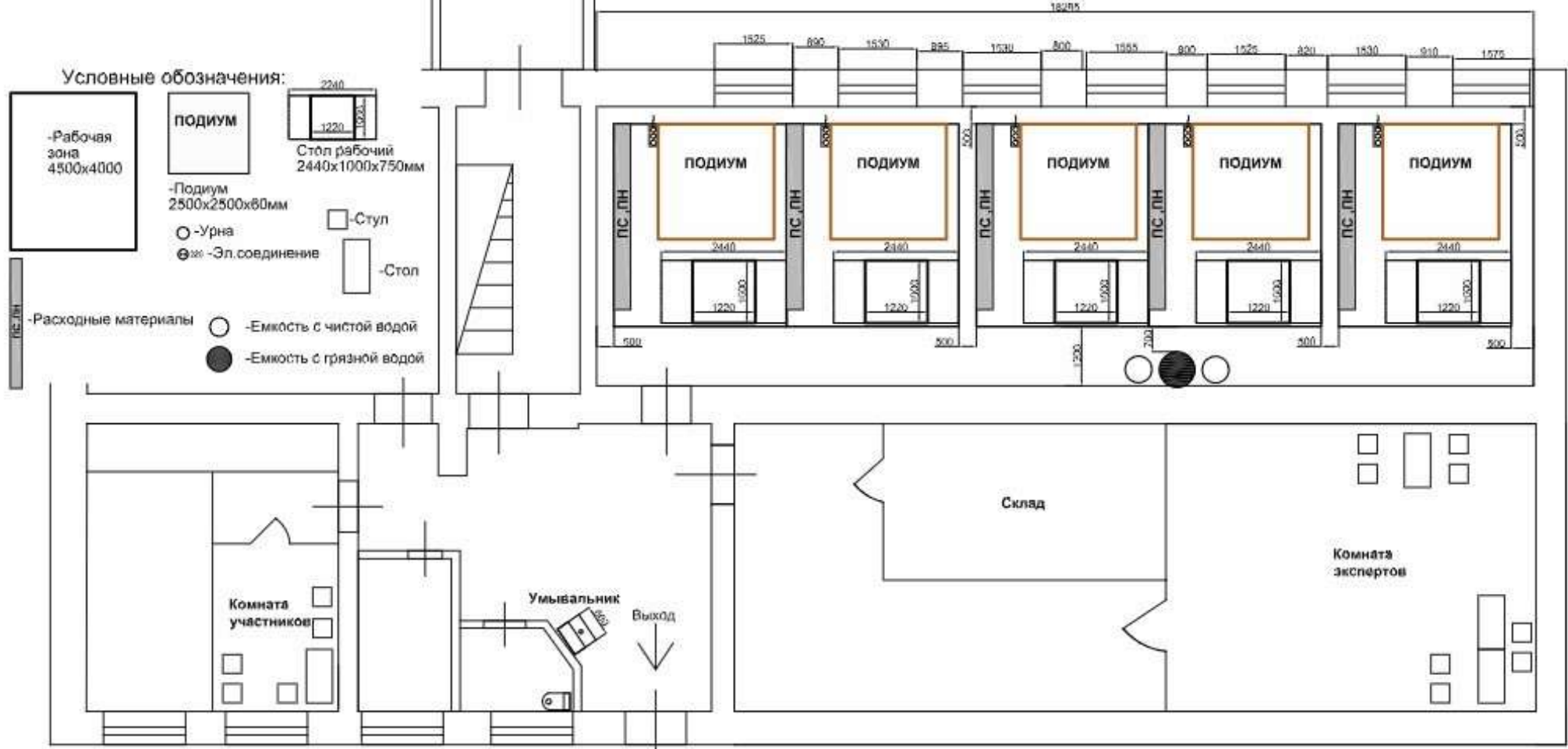
План застройки по компетенции "Сухое строительство и штукатурные работы"
